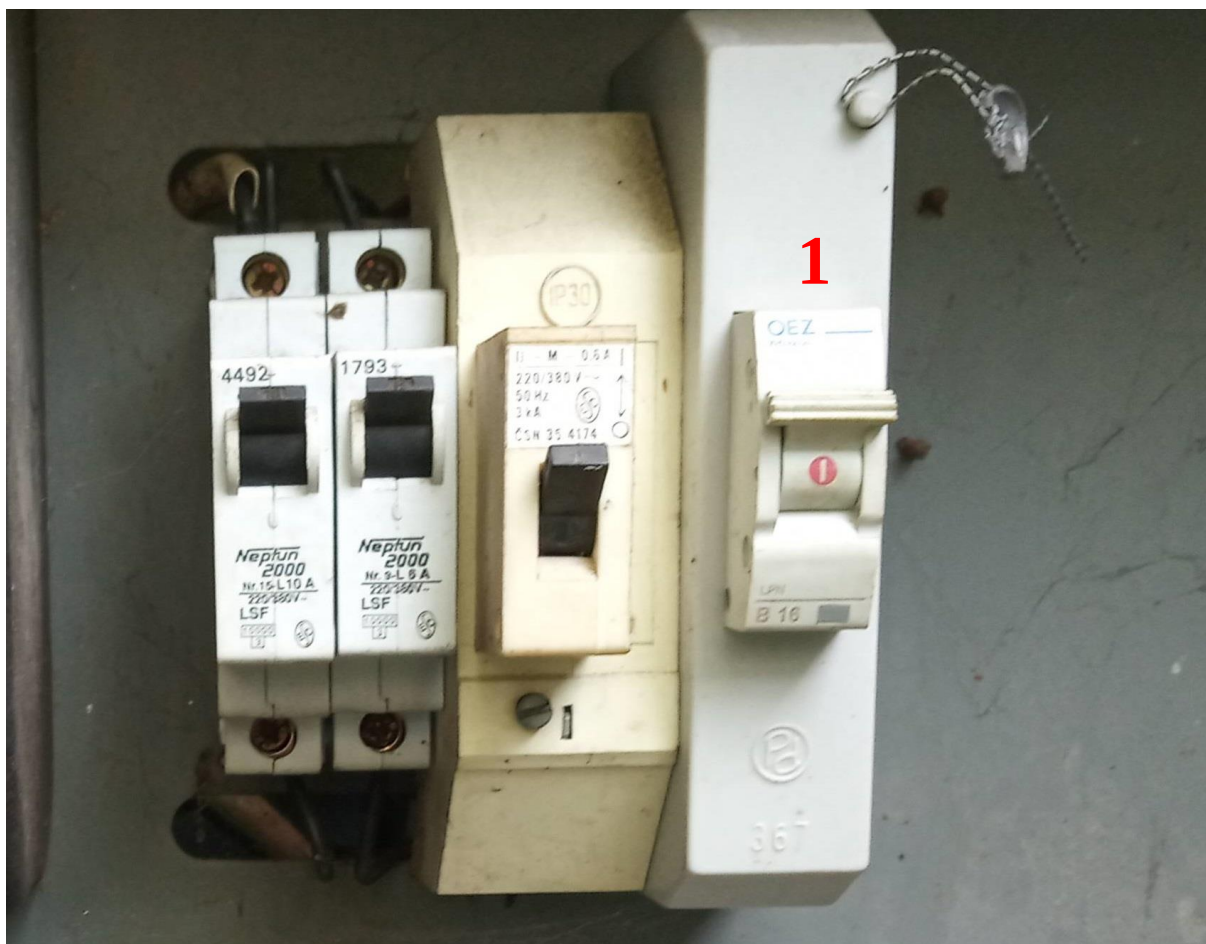
Obr. 4: Číslování větví na RVO-2, dle číslování v pasportu
