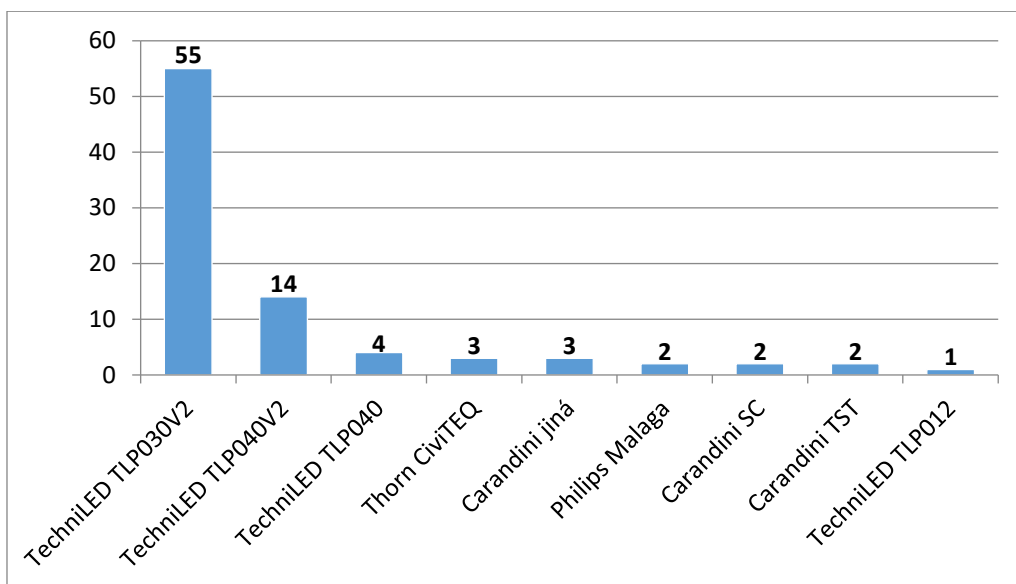
Obr. 5: Zastoupení jednotlivých typů svítidel v obci Kovalovice
