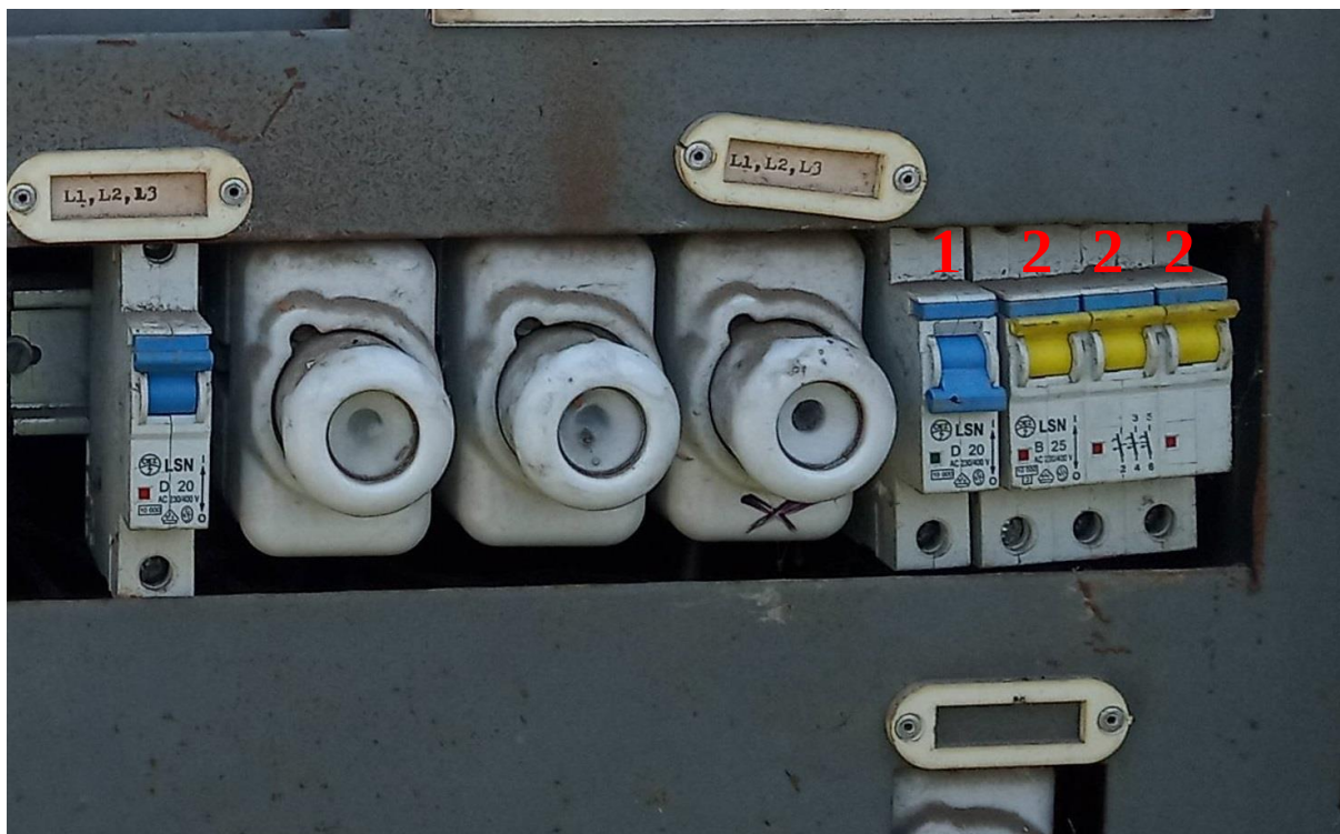
Obr. 3: Číslování větví na RVO-1, dle číslování v pasportu
